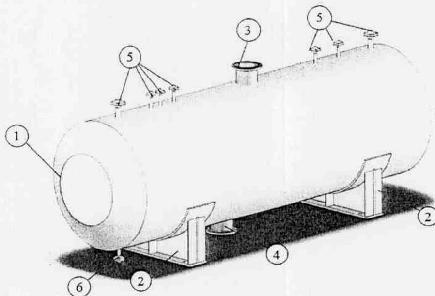
Рис. 96.1. Горизонтальная емкость для жидкости
