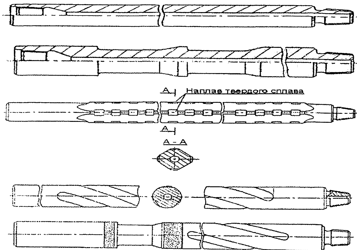
Рис. 107.1. Внешний вид утяжеленных бурильных труб
