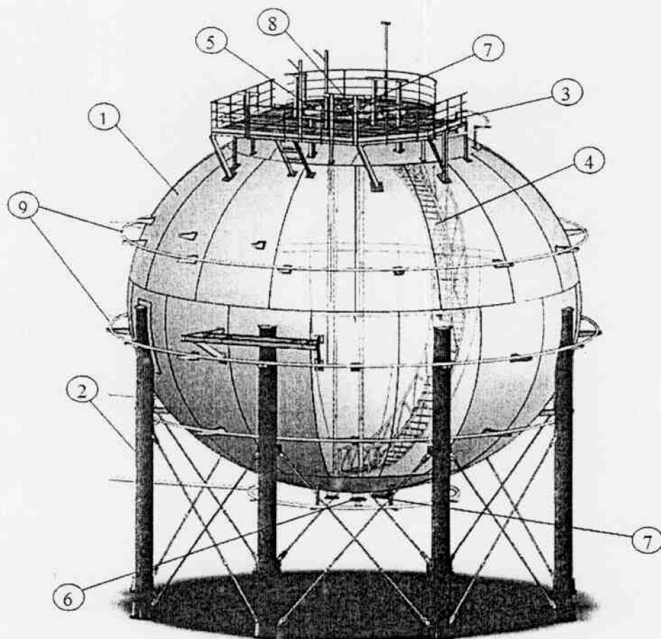
Рис. 97.2. Типовая схема шарового резервуара
