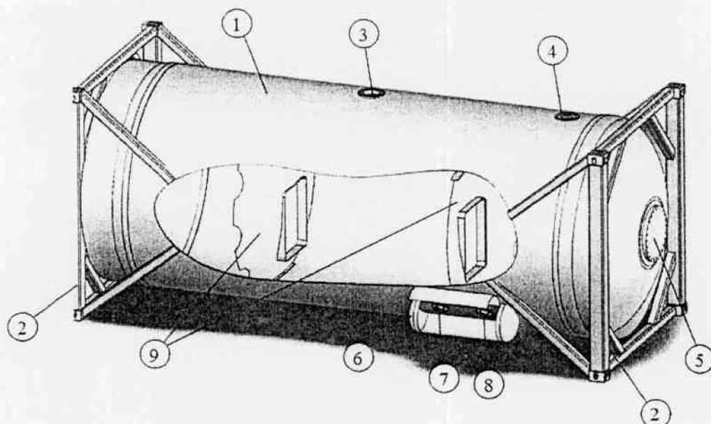
Рис. 97.1. Емкость для хранения сжиженных газов под давлением
