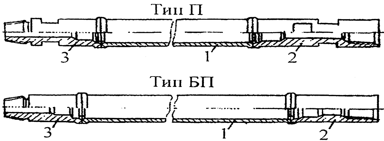
Рис. 107.3. Внешний вид бурильных труб
