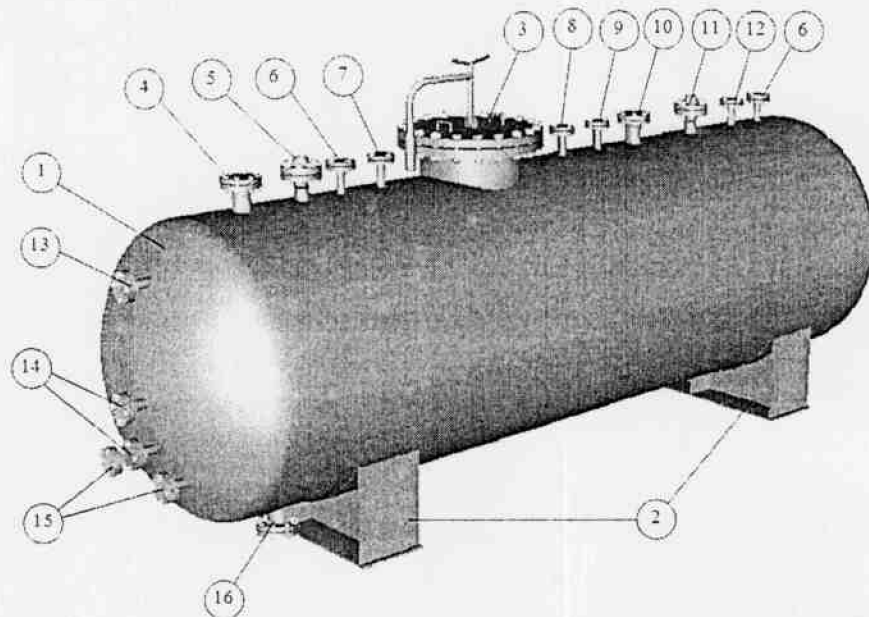
Рис. 95.3. Типовая емкость малой вместимости
