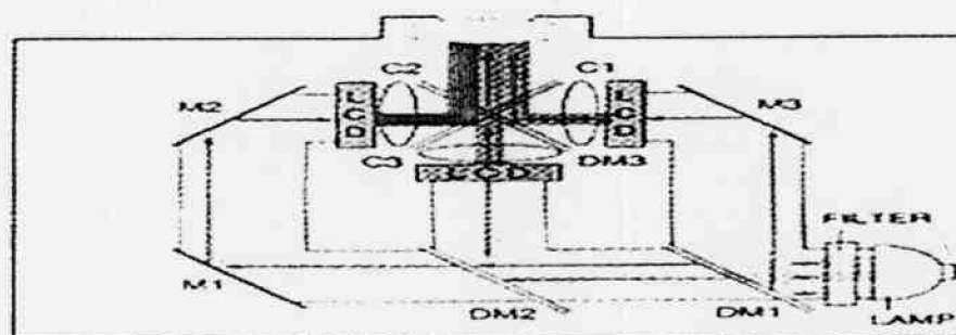
Рис. 135.1. Конструкция и принцип работы трехматричного LCD-проектора
