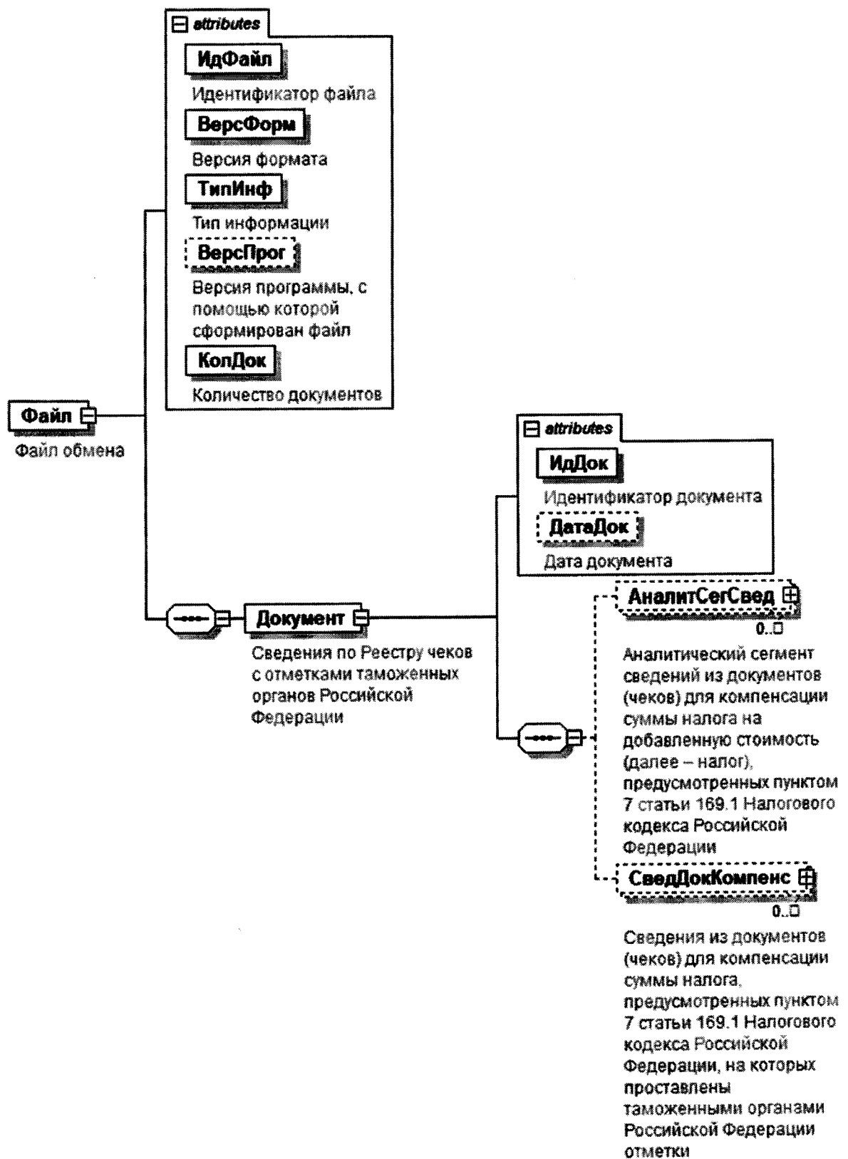
Рис.1. Диаграмма структуры файла обмена
