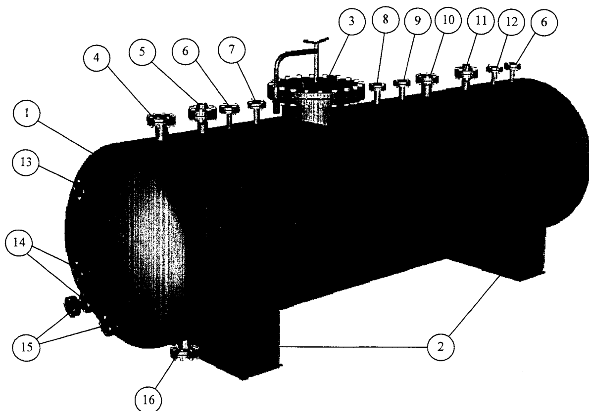
Рис. 37 Типовая емкость малой вместимости
