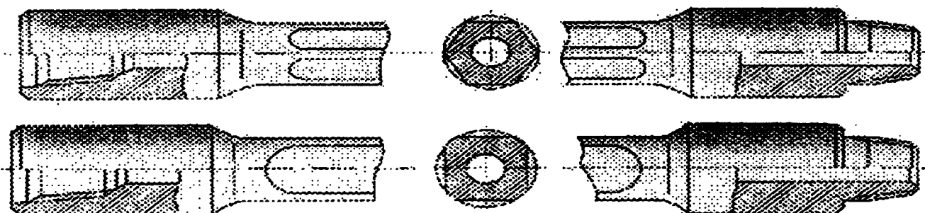
Рис. 29 Внешний вид ведущих бурильных труб
