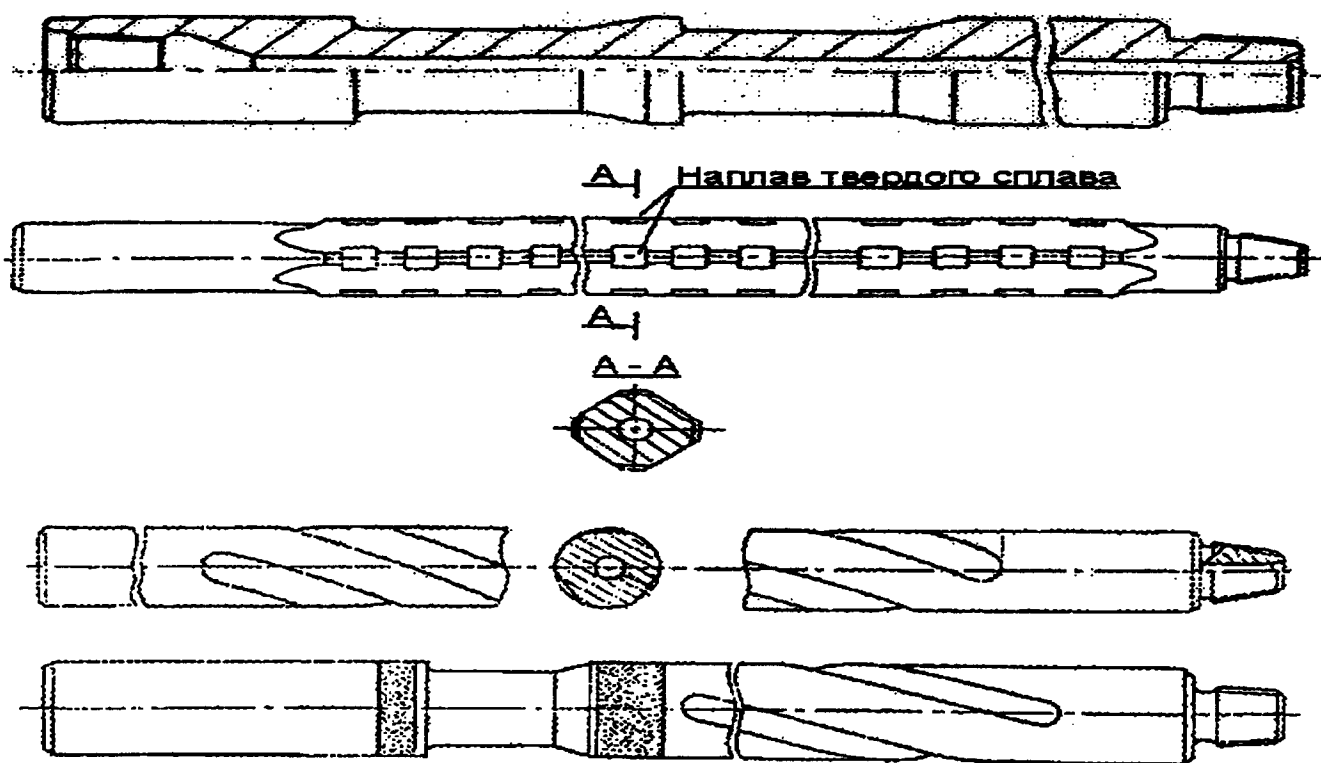
Рис. 28 Внешний вид утяжеленных бурильных труб
